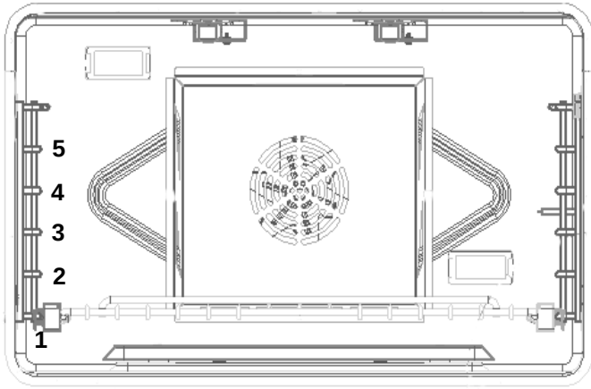
Figura 29: Hornilla principal y posiciones de las rejillas
