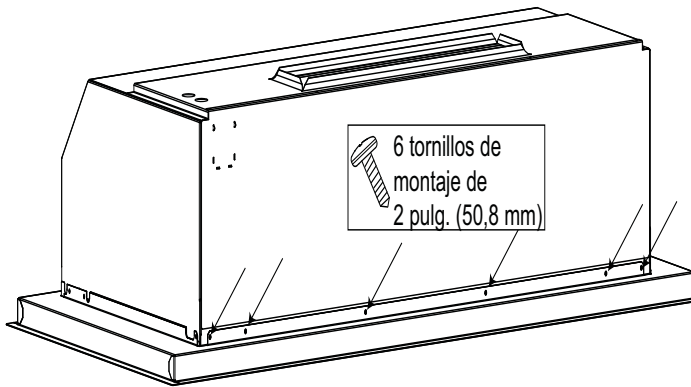
Figura 36: Tornillos traseros de los modelos VCIB
