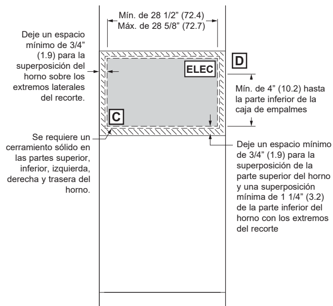
VISTA FRONTAL DE LA INSTALACIÓN
