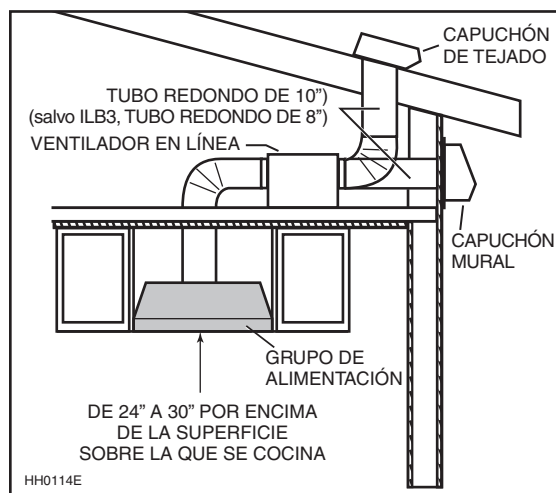
INSTALACIÓN HABITUAL DE LOS TUBOS CON UN VENTILADOR EN LÍNEA MODELO ILB3, ILB6, ILB9 o ILB11 DE LA SERIE CP57E (UBICACIÓN DEL VENTILADOR SÓLO A MODO DE EJEMPLO)
