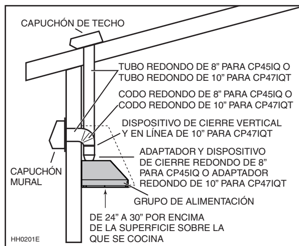
INSTALACIÓN HABITUAL DE LOS TUBOS, MODELOS DE LA SERIE CP55IQ (UN SOLO VENTILADOR INTERIOR) o CP57IQT (DOBLE VENTILADOR INTERIOR)
