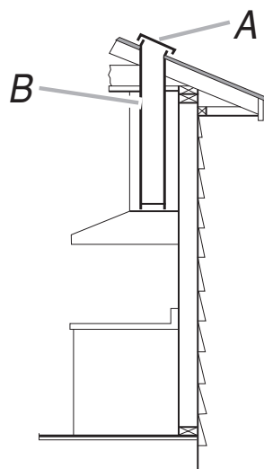
A. Bouche de décharge sur toit B. Coude de ventilation métallique rectangulaire 90° de 3 1/4 po x 10 po (8,3 cm x 25,4 cm)
